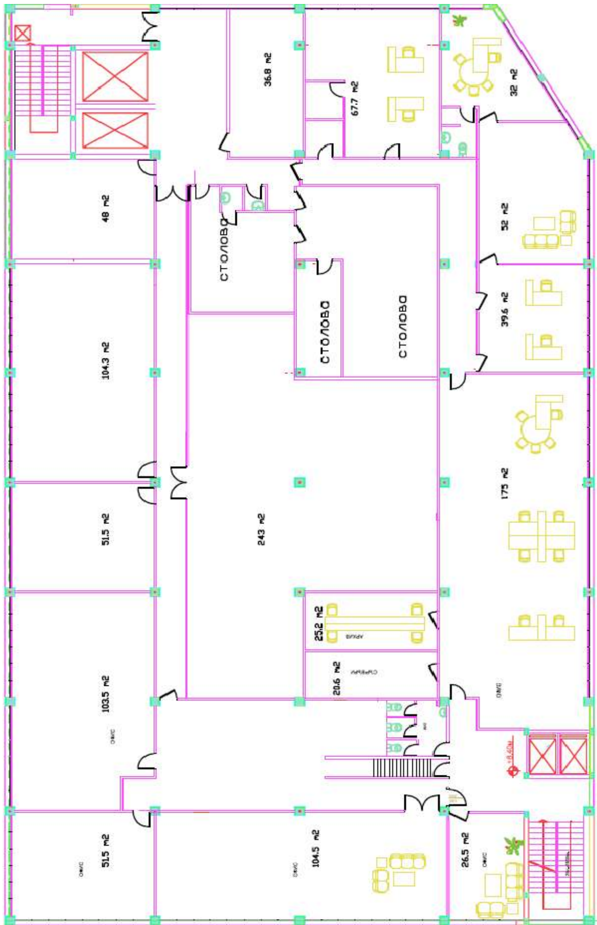
Technologiezentrum Sofia Grundrissplan - 1500 qm, M1:100
